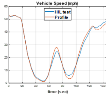
(d) Vehicle Speed (mph)
